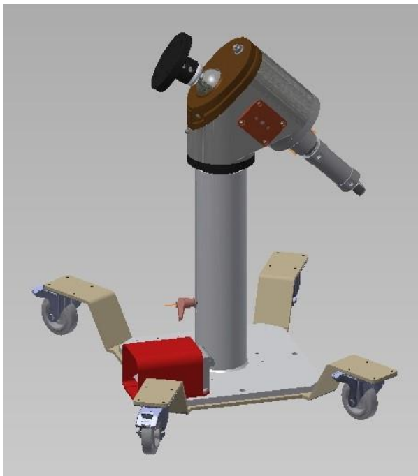
Abbildung 3 Simon Standard mit Fahrwerk APO Anlagenbau GmbH
